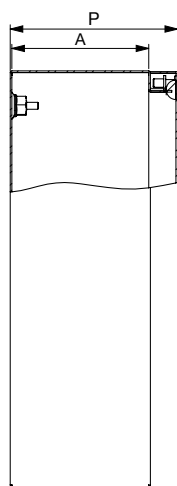
Vista laterale
